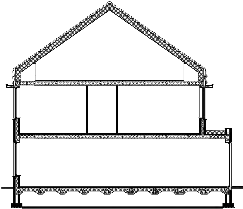
aanzicht zijgevel 1:100
